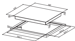
INSTALLAZIONE FILO TOP FLUSH FIT INSTALLATION
