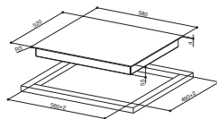
INSTALLAZIONE STANDARD STANDARD INSTALLATION
