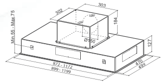
Uscita aria orientabile in 4 posizioni Air outlet adjustable in 4 positions
